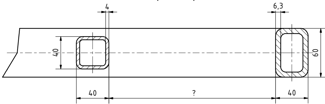
A-A ( 1 : 2 )
