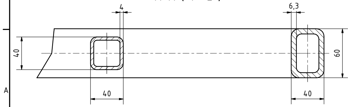
A-A ( 1 : 2 )
